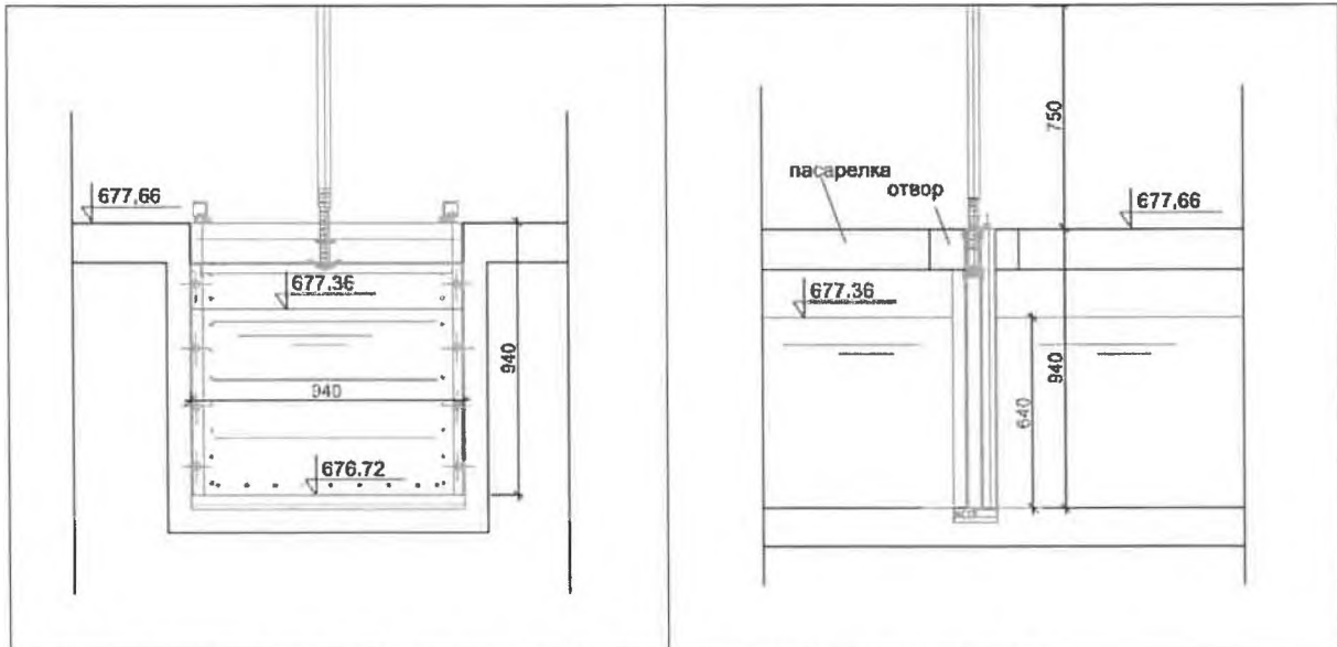
фиг. 7 Саваци от първа група – за каналите за избистрена вода
