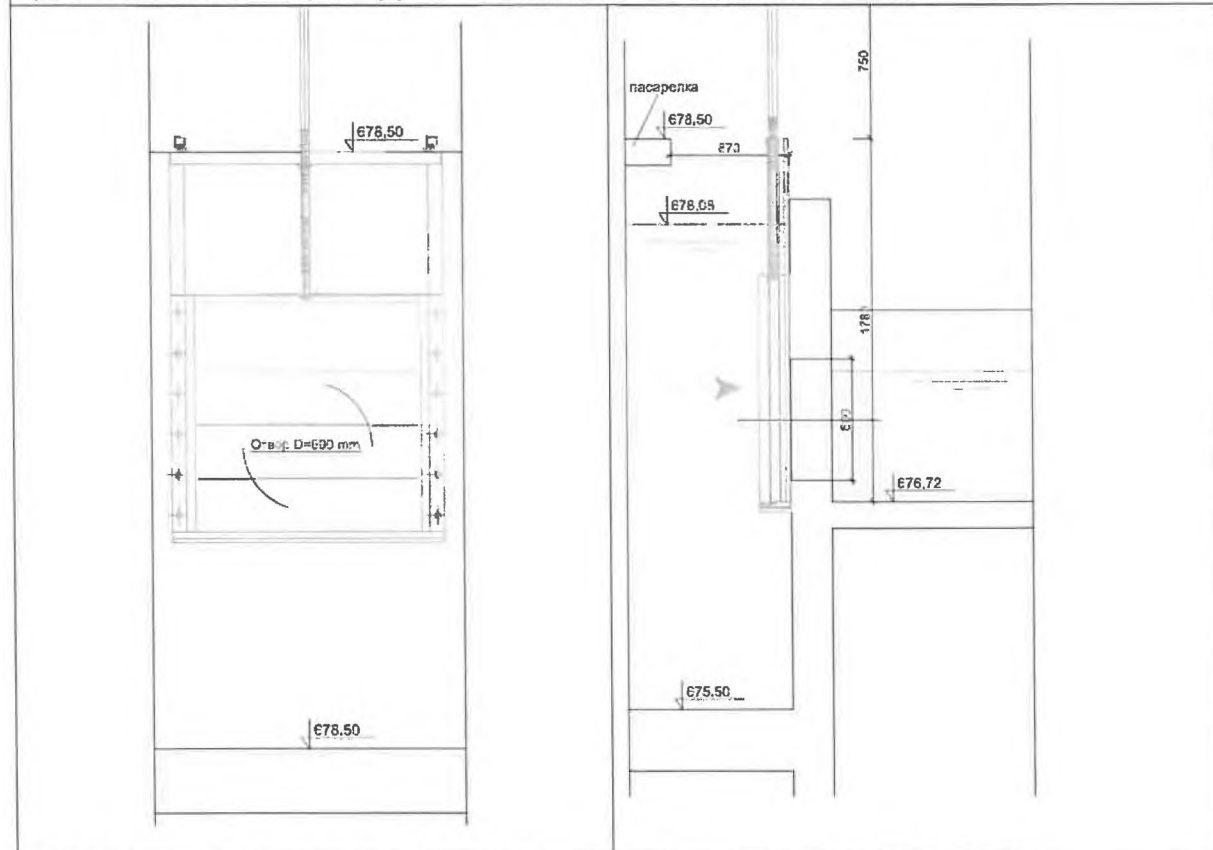
фиг.8 Саваци от втора група – за началото на байпасиращите канали
