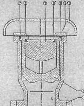
Воздушник DN 100 - DN 200
