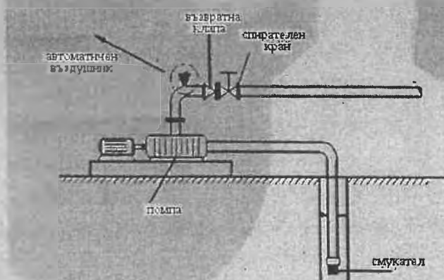
Примерна схема за разполагане на въздушник при обслужване на помпа
