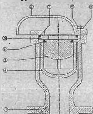
Воздушник DN 40 - DN 80
