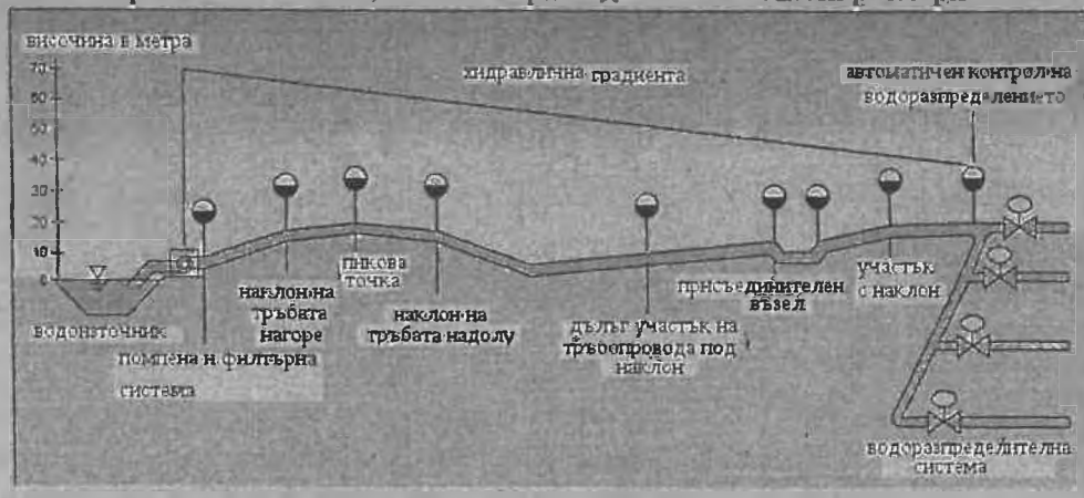
Примерна схема за разполагане на въздушници при монтаж във водоразпределителна система
