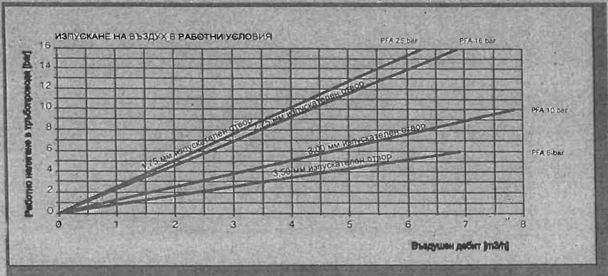
Диаграма на дебитно изпускателния потенциал на въздушник еднодействащ
