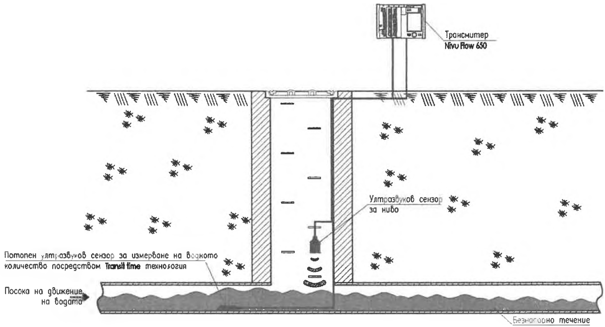
Схема 3 – примерно измерва на водно количество в непълен водопровод
