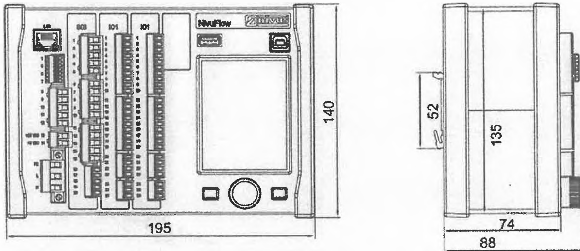
Схема 1 – размери на трансмитера
