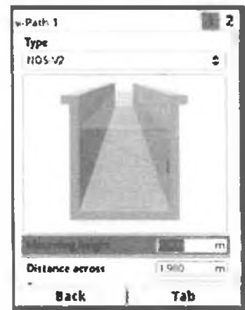
Размери на профила
